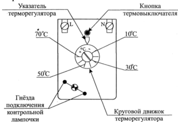
Рисунок 2 – Вариант лицевой панели термостата
